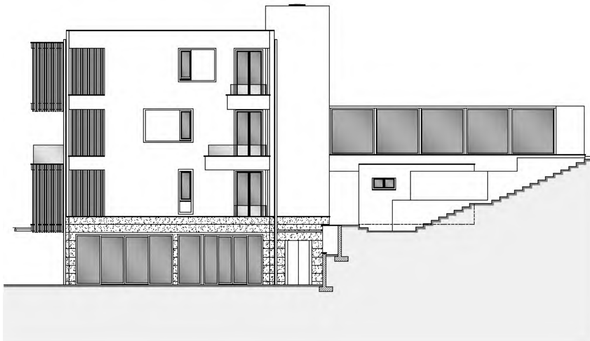
Slika 15. Budući vanjski izgled objekta Smiljka – jugoistočno pročelje
