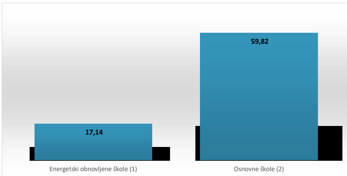
Slika 12. Grafički prikaz specifične potrošnje peleta (kWh/m²) u sektoru zgrada Primorsko-goranske županije po vrstama objekata
