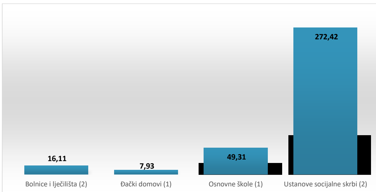
Slika 10. Grafički prikaz specifične potrošnje UNP (kWh/m 2 ) u sektoru zgrada Primorsko-goranske županije po vrstama objekata
