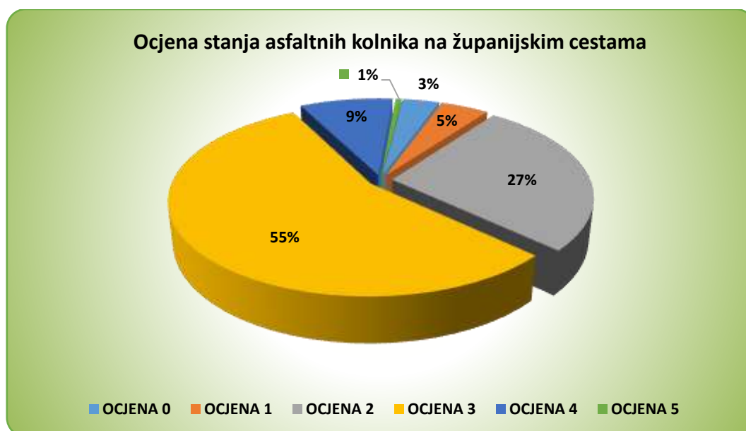
Grafikon 6. Ocjena stanja asfaltnih kolnika na županijskim cestama
