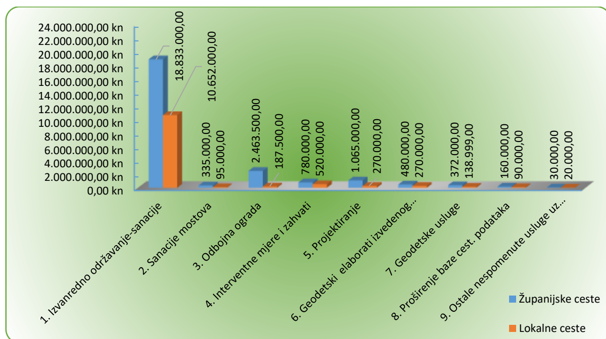
Grafikon 10. Skup mjera i radnji izvanrednog održavanja
