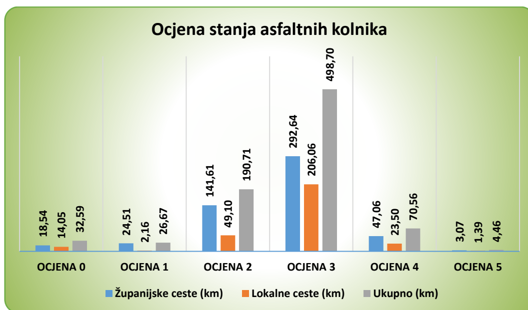
Grafikon 5. Ocjena stanja asfaltnih kolnika
