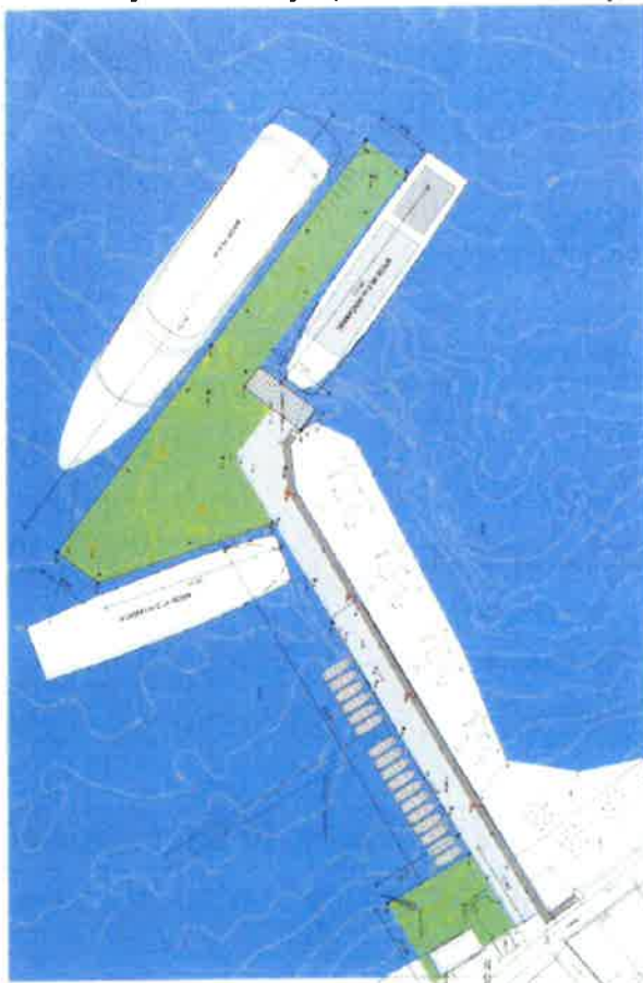
Slika 2. Novo planirane stanje luke Unije (zeleno označeno područje izgradnje)
