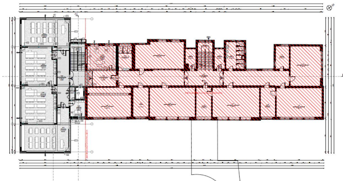
Skica 11: Tlocrt drugog kata novog stanja Osnovne škole „Dr. Andrije Mohorovičića“
