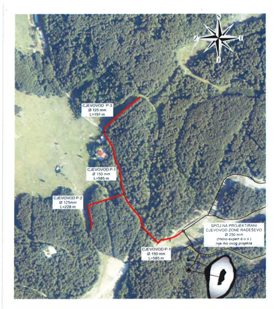
Slika 2. Sustav zasnježenja staza Baby lift i Pribeniš
