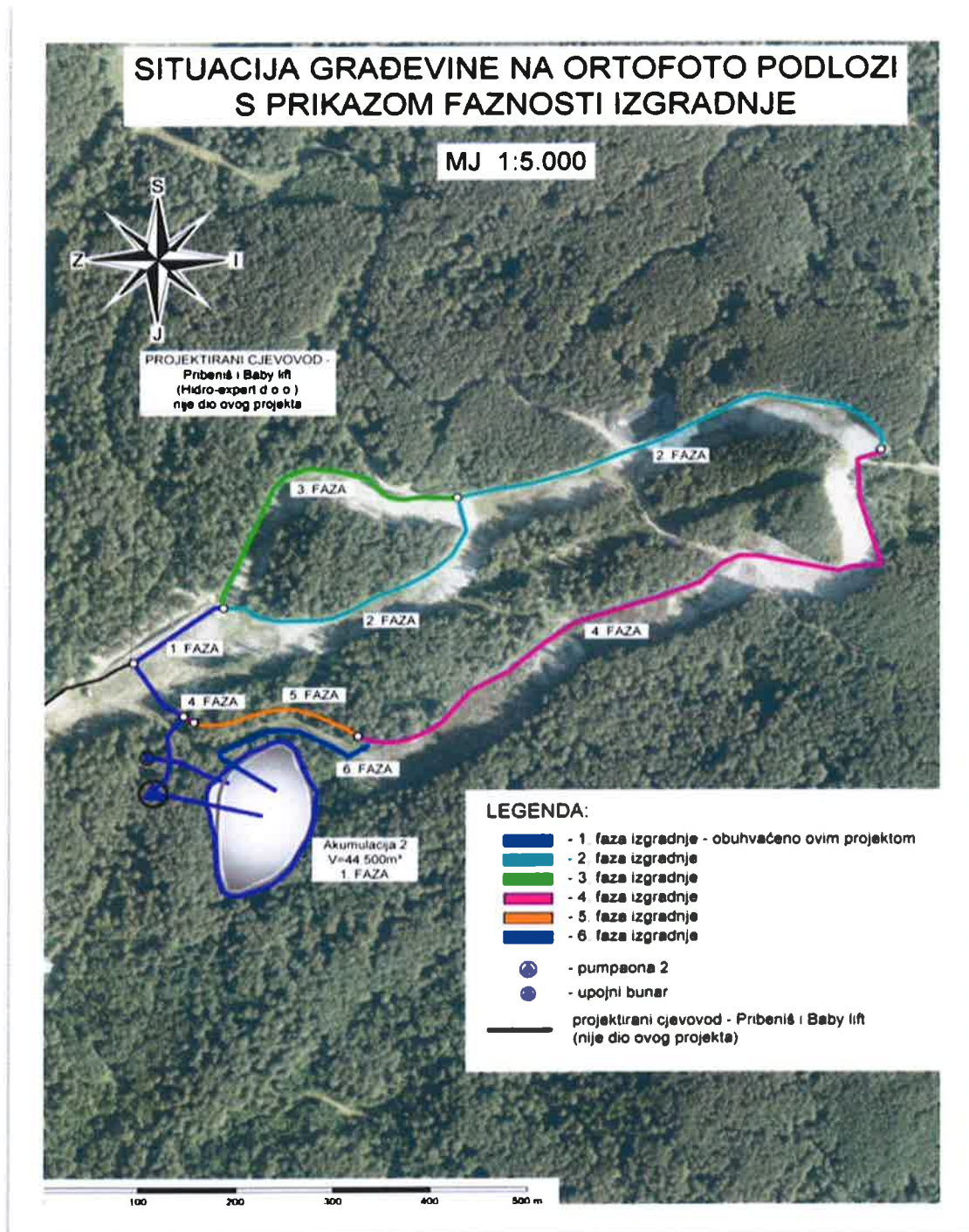
Slika 1. Sustav zasnježenja Radeševo
