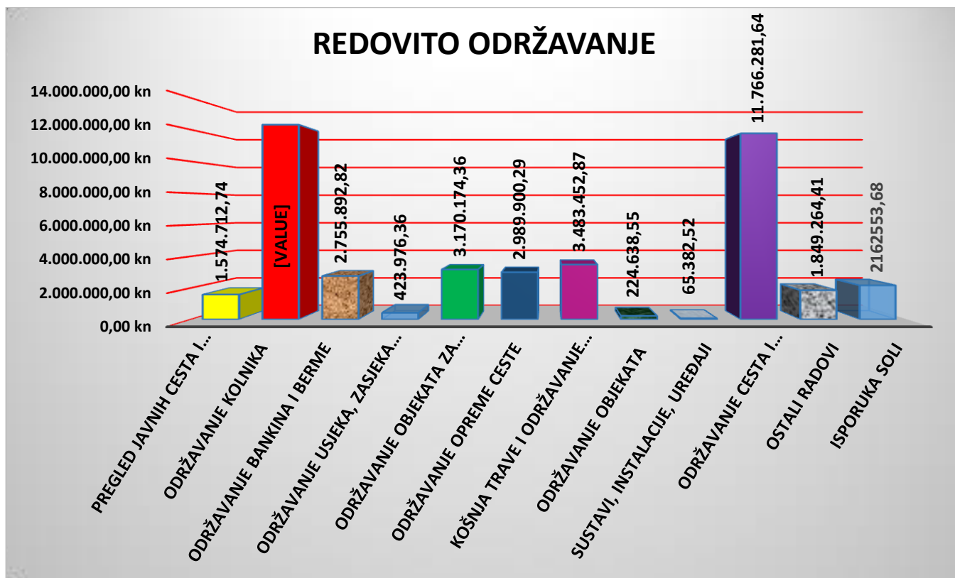
Grafikon 5 Vrste i vrijednosti izvedenih radova redovnog održavanja cesta bez obzira na kategoriju cesta
