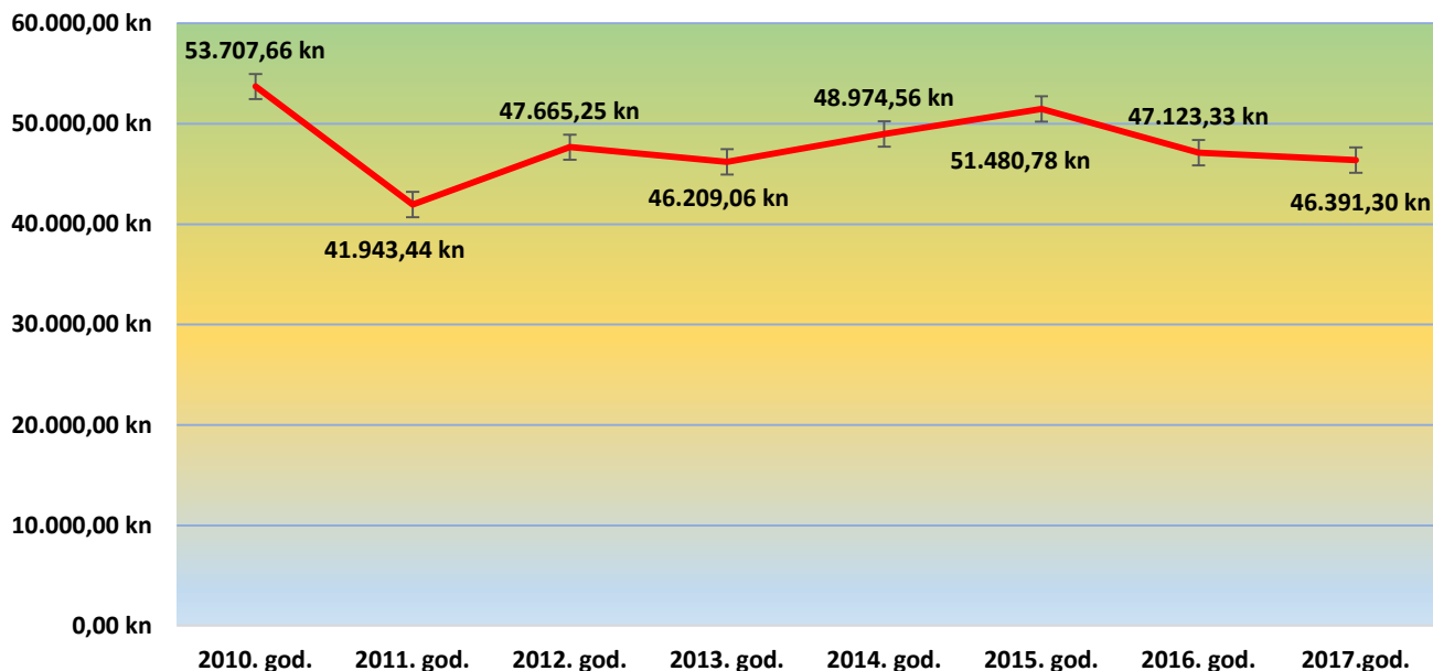
Grafikon 12 Pregled ulaganja u redovito održavanje županijskih i lokalnih cesta po kilometru (2010.god.-2017.god.)
