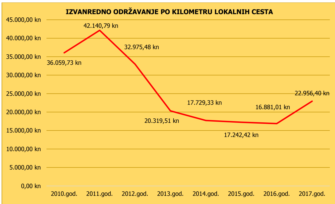
Grafikon 24 Pregled ulaganja u izvanredno održavanje lokalnih cesta po kilometru (2010.god.-2017.god.)
