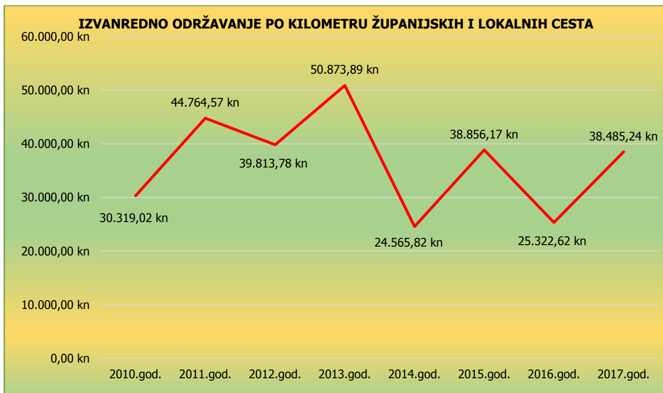
Grafikon 25 Pregled ulaganja u izvanredno održavanje županijskih i lokalnih cesta po kilometru (2010.god.-2017.god.)
