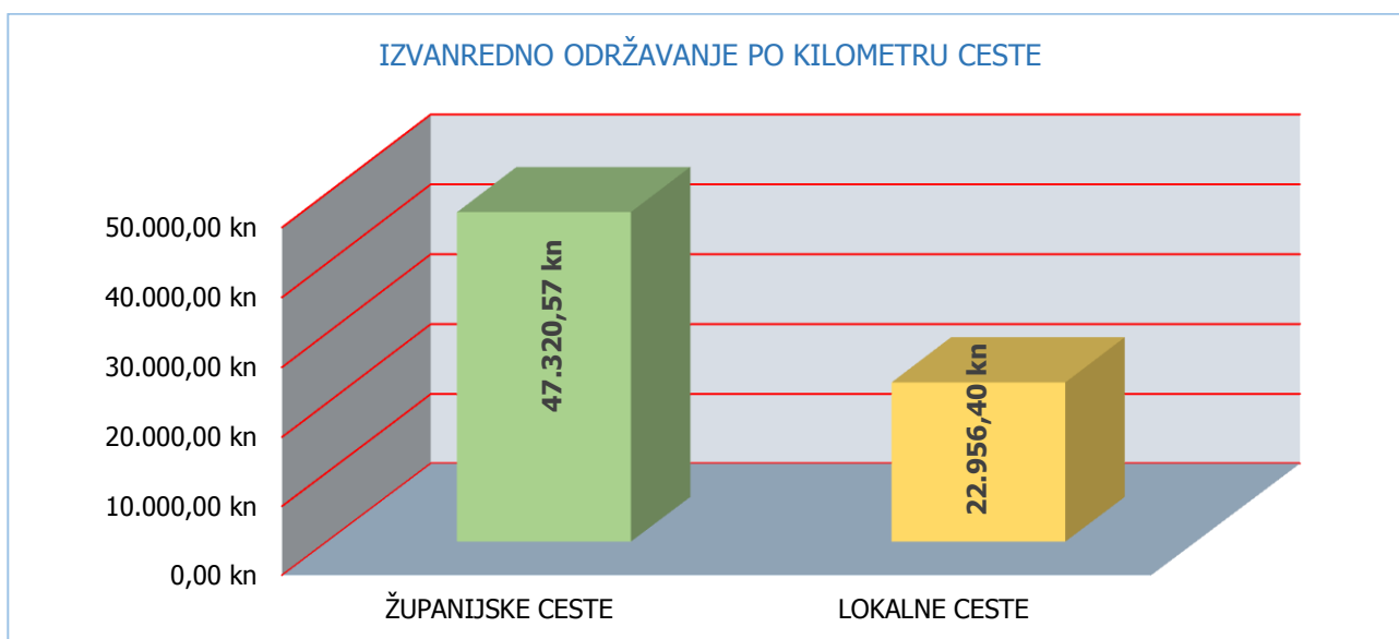
Grafikon 20 Realizacije izvanrednog održavanja po kilometru obzirom na kategoriju cesta
