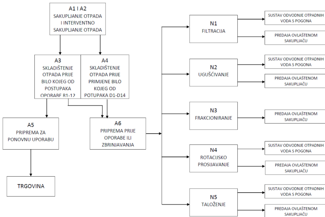
Slika 1. Shema tehnoloških procesa gospodarenja neopasnim otpad u pogonu Urinj
