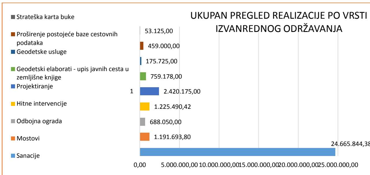
Grafikon 17 - Grafikon realizacije izvanrednog održavanja županijskih cesta po vrsti radova/usluga
