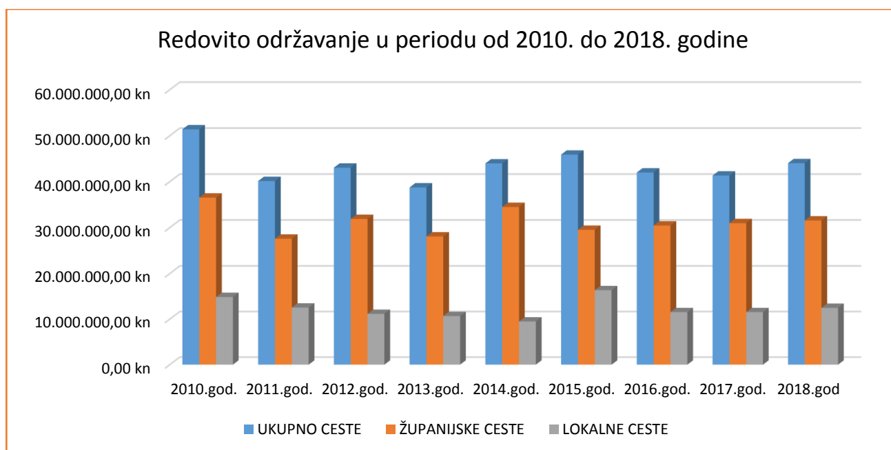
Grafikon 8 - Grafikon realizacije redovitog održavanja ukupno te obzirom na kategoriju cesta
