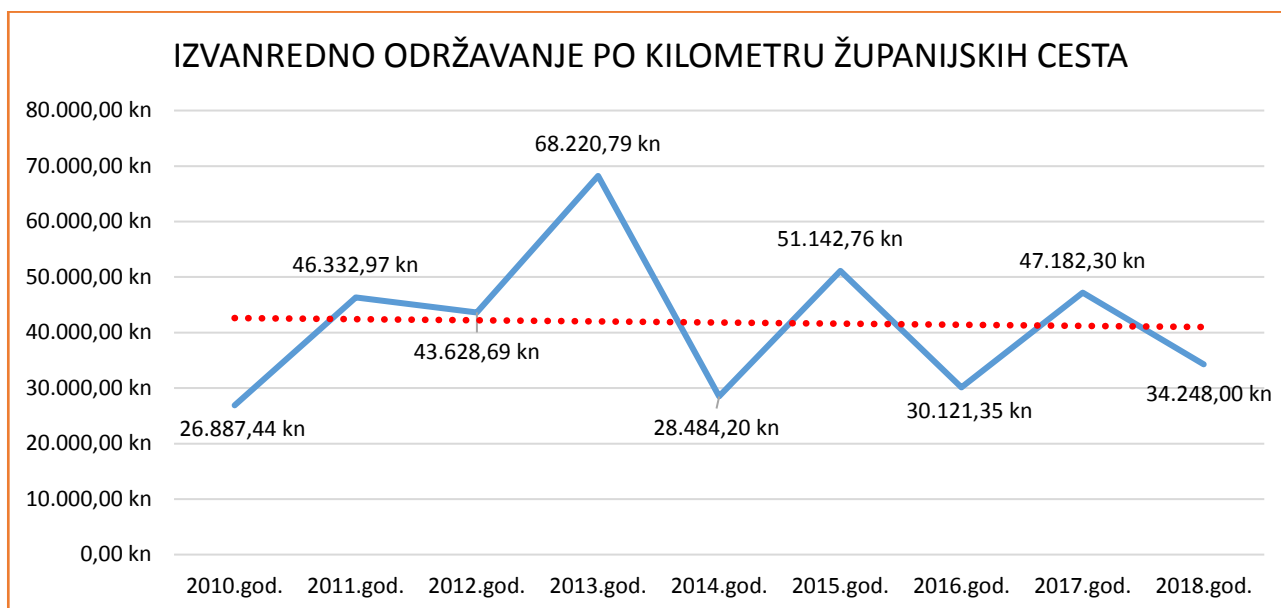
Grafikon 23 - Pregled ulaganja u izvanredno održavanje županijskih cesta po kilometru (2010.god.-2017.god.)
