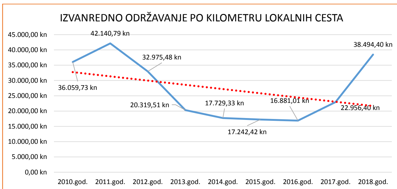
Grafikon 24 - Pregled ulaganja u izvanredno održavanje lokalnih cesta po kilometru (2010.god.-2017.god.)
